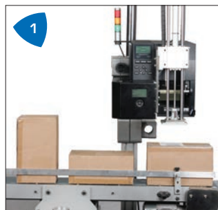
1 Etichettatura in movimento di prodotti di diverse dimensioni fino a 30 etichette al minuto.
